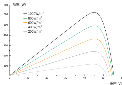
功率 - 电压曲线 (625W)
