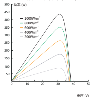
功率 - 电压曲线 (445W)
